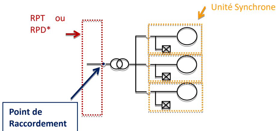
Figure 1 - Description du périmètre d'une Unité synchrone
