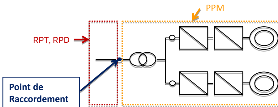
Figure 2 - Description du périmètre d'une Unité non synchrone
