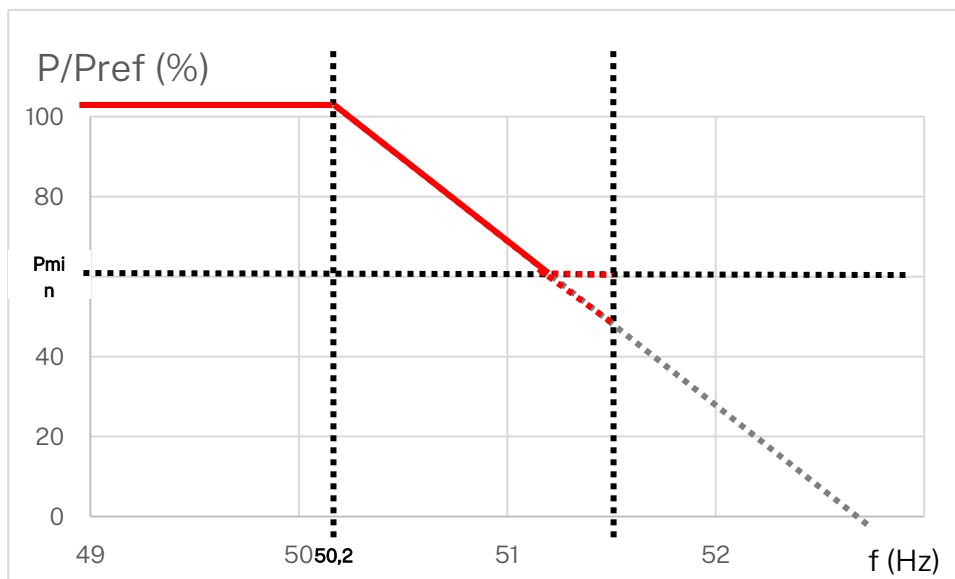
Figure 4 - Loi de régulation de la puissance en fonction de la fréquence pour un statisme de 5 % et P_{min} = 60 \% * Pref
