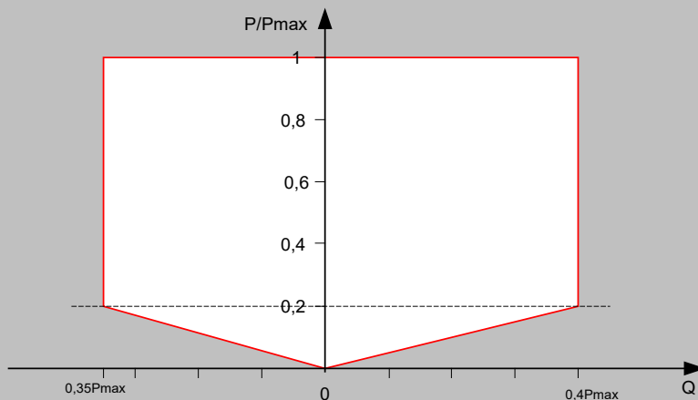
Figure 2 - Diagramme [P, Q] requis au PdR pour les Unités de Production de type A et B (en HTA et BT)
