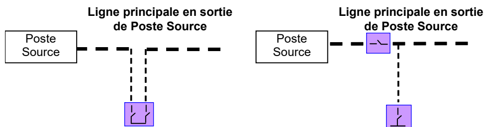
Figure 16 - Interrupteur pour faciliter la réalimentation en cas de mise hors tension du Poste Source
