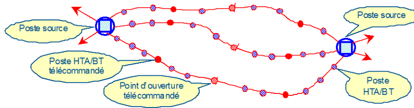
Figure 7 : exemple de structure en coupure d'artère
