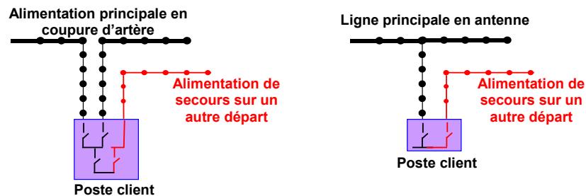
Figure 19 - Schémas d'alimentation pour une alimentation de secours
