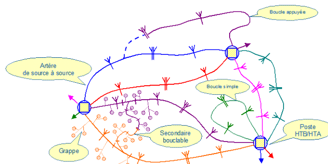
Figure 9 : structure de réseau rural
