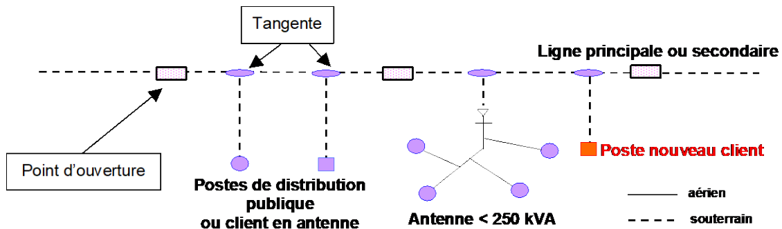
Figure 14 - Illustration de la règle de deux tangentes maximum entre deux points d'ouverture
