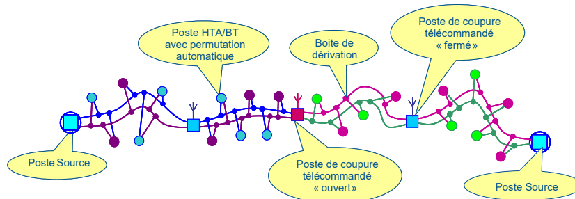
Figure 8 : exemple de structure en double dérivation
