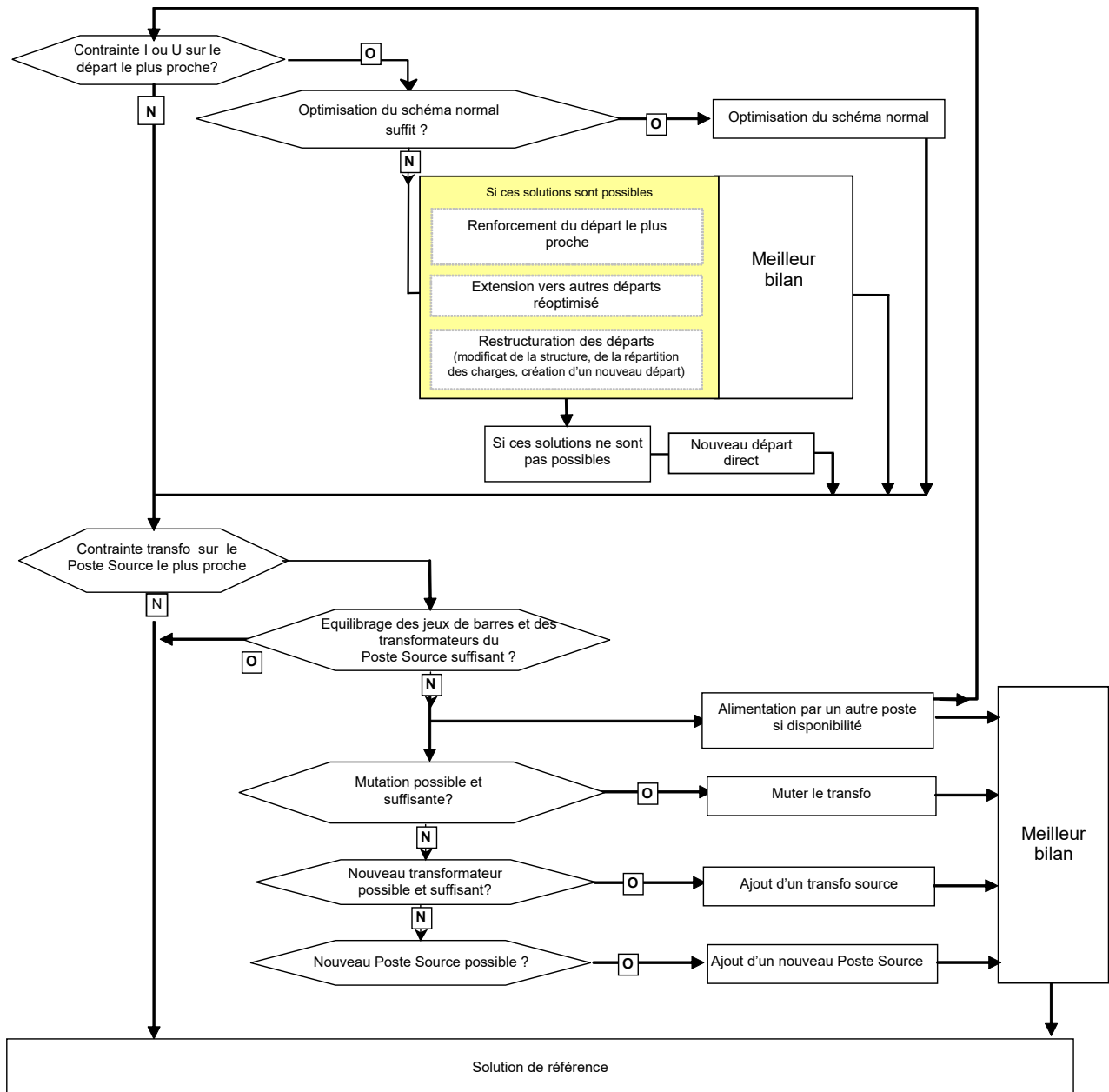
Figure 13 - Principe de levée de contrainte après raccordement
