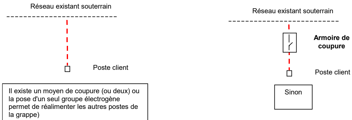
Figure 18 - Moyen de séparation d'un poste de livraison sur un réseau souterrain
