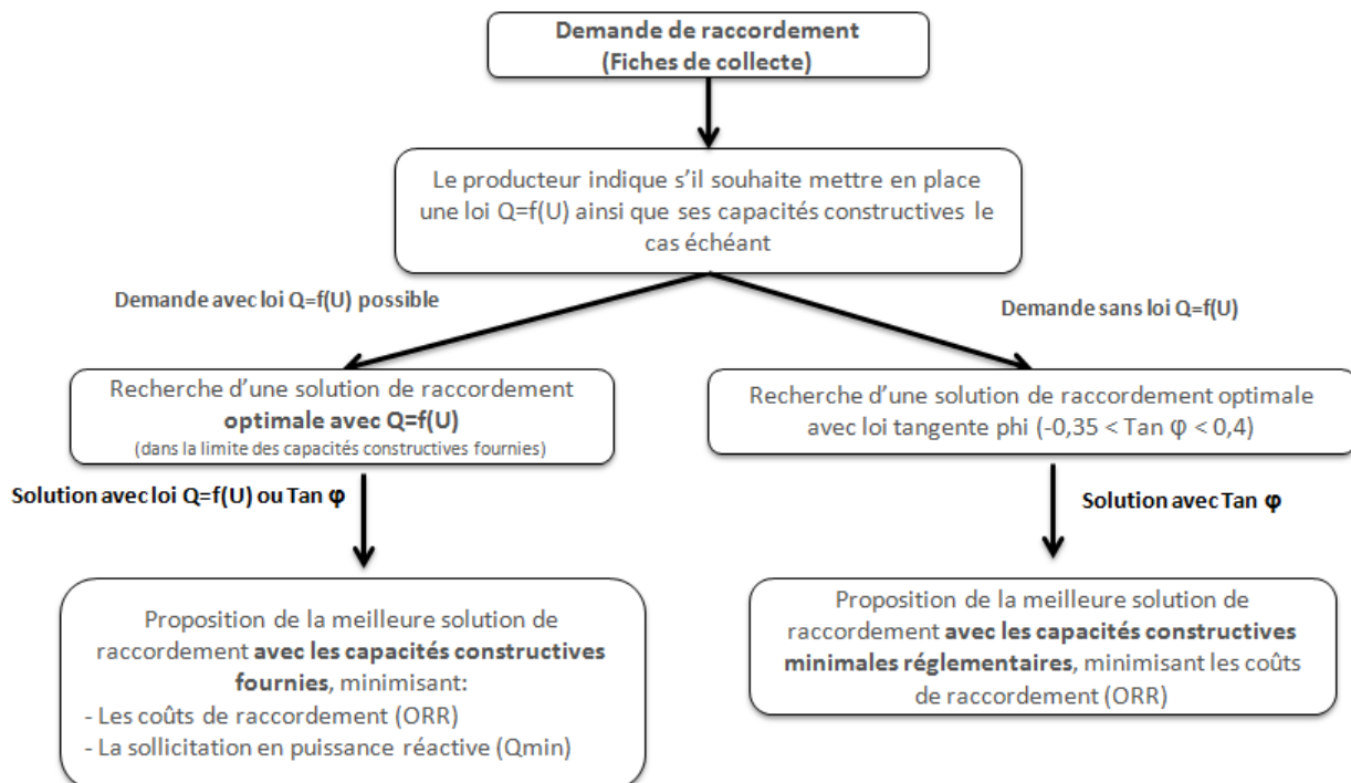
Principe de l'étude de raccordement
