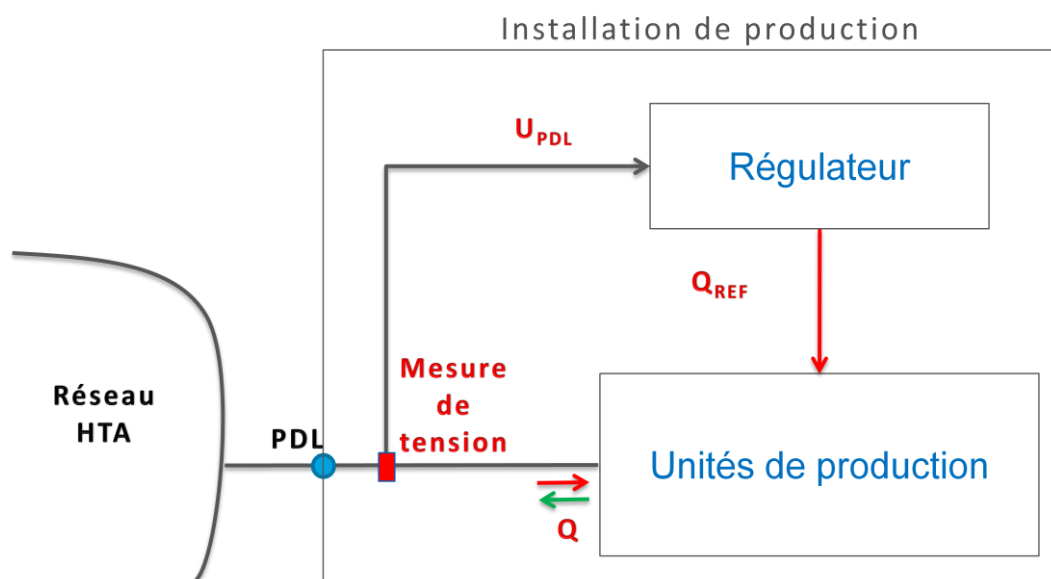
Principe de la régulation locale Q=f(U) pour une Installation de Production raccordée en HTA
