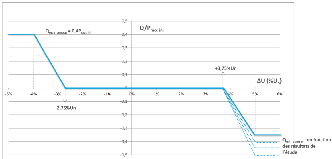
Loi de régulation locale Q=f(U)
